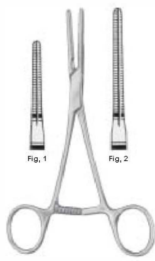
COOLEY ----- Gerade Abgewinkelt Straight Angled Recta Angular Fig.1 14,0 cm 90080-0-14 Fig.1 14,0 cm 90080-1-14 Fig.2 16,0 cm 90080-0-16 Fig.2 16,0 cm 90080-1-16
